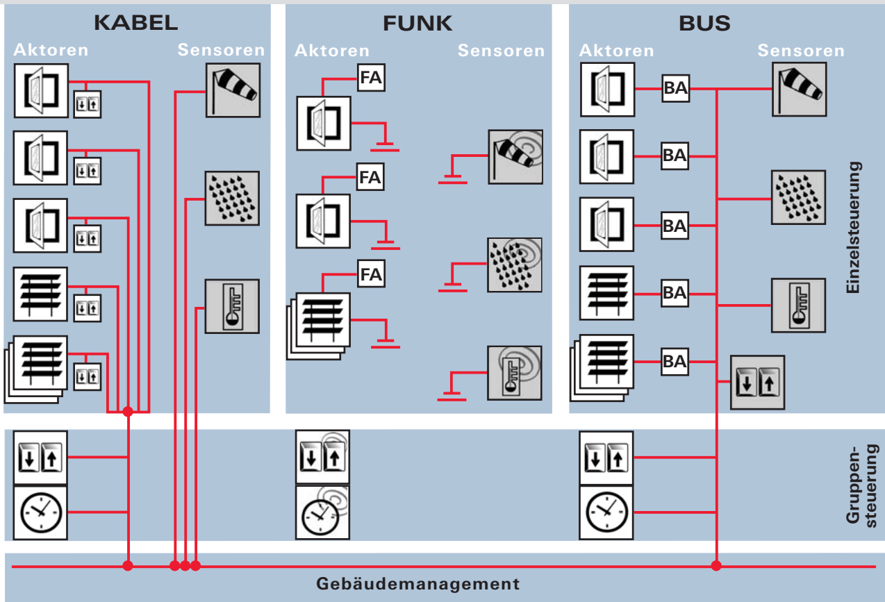
Roto E-Tec Drive: Ermöglicht das bedarfsgerechte, kontrollierte Belüften von einzelnen Räumen und kompletten Gebäuden
